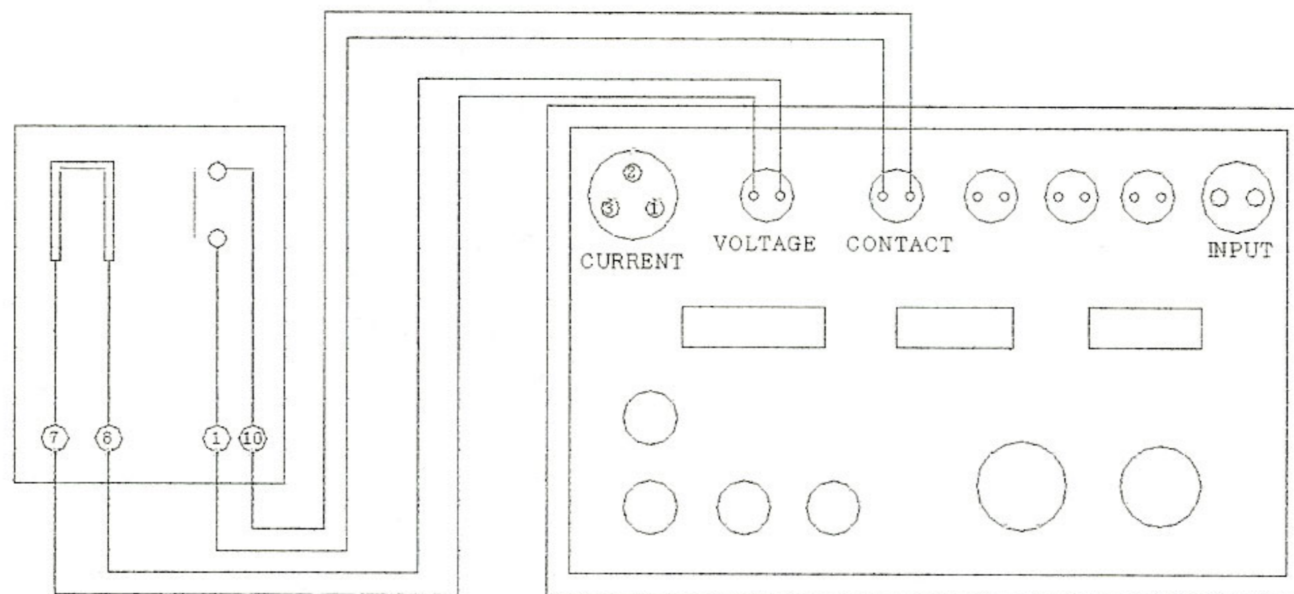
<계전기 시험기>
